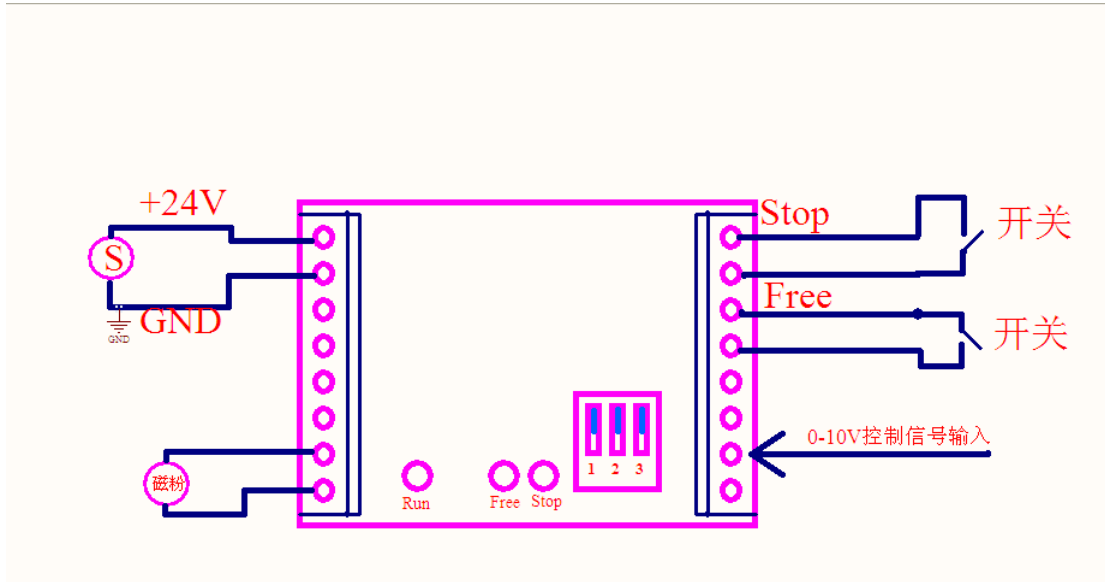
0-10V 信号输入控制方式接线图
