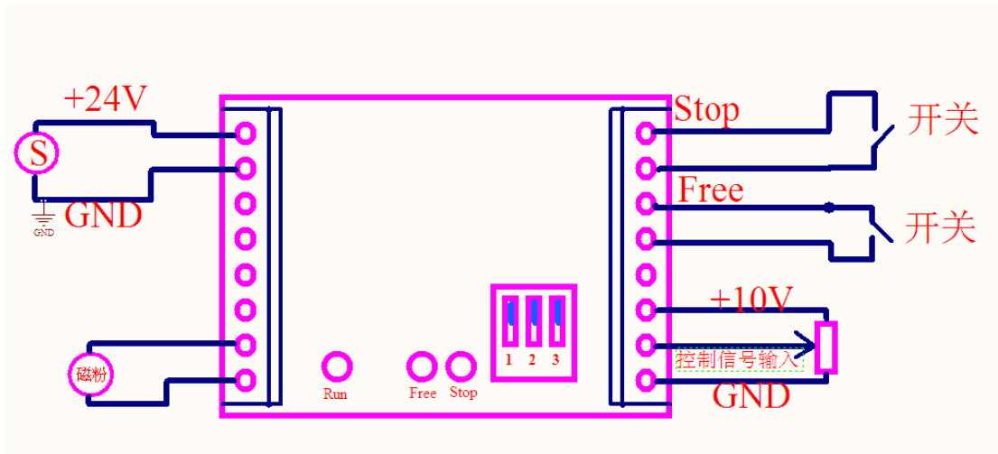
电位器控制方式接线图
